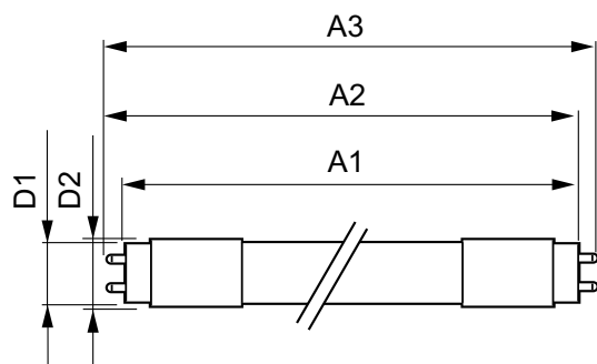
LEDtube HF 1500mm HO 25W 840 T8
