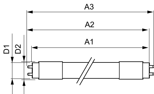
TLED 5ft 20W-58W 3100lm 160D 6500K G13ND
